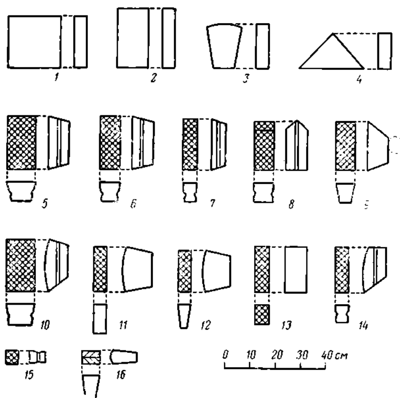
Рис. 3. Золотоордынские мавзолеи у Ессентуков 1—4 — строительные кирпичи; 5—16 облицовочные кирпичи
