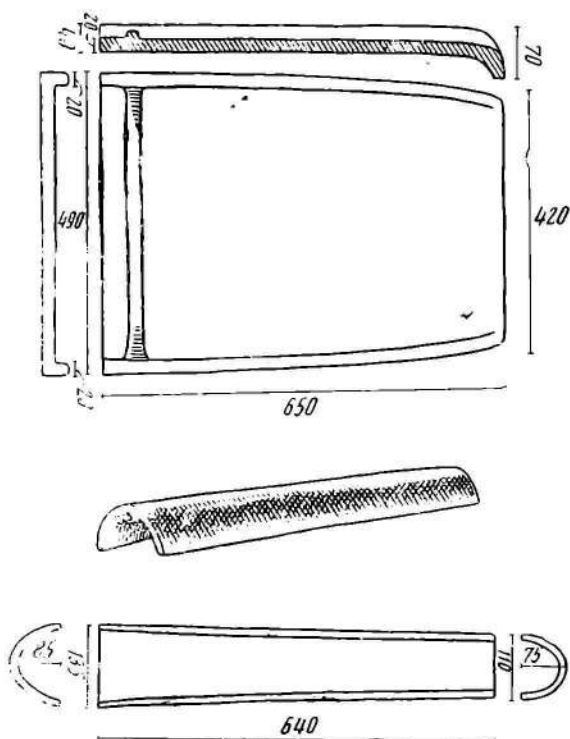
Рис. 2. 1 — плоская черепица (солен). II — первая половина I в. до н. э.; 2 — желобчатая черепица (калиптер). II в — первая половина I в. до н. э.
