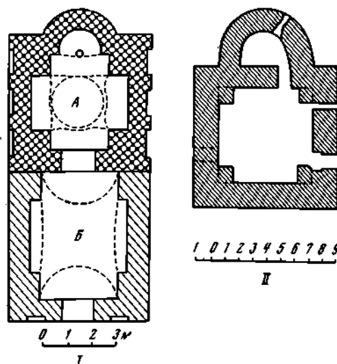
Рис. 12. Сопоставление планов Боянской церкви и подклета Благовещенского собора.
