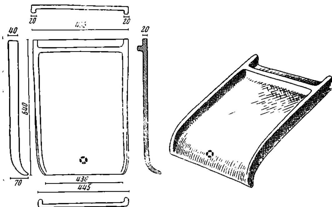
Рис. 1. Плоская черепица (солон) с клеймом. II — первая половина I в. до н. э.
