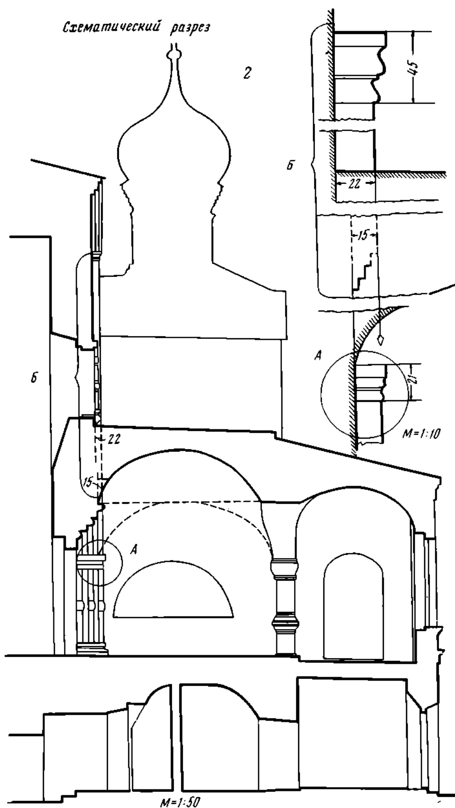
2,6 — схематический поперечный разрез южной галереи (чертеж)
