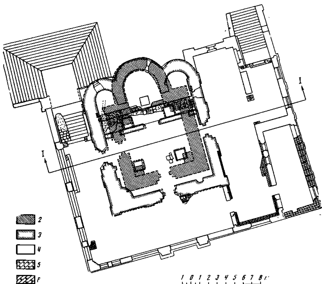
Рис. 5. Схема реконструкции плана первого этажа Благовещенского собора. 2 — II строительный период, конец XIV в.; 3 — III период, 1416 г.; 4 — IV период, 1484—1489 гг.; 5 — V период, 1564; 1572 гг.; 6 — кладка XIX в. Архитектор В. И. Федоров, 1972 г. (условное обозначение 1 — см. рис. 6)
